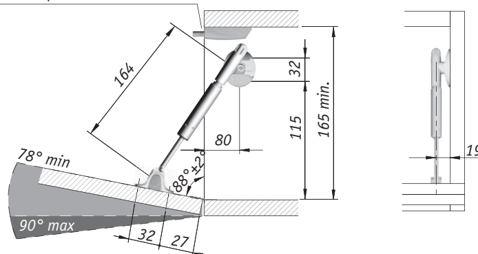
Толкатель K-PUSH TECH короткий с магнитом врезной или накладной
