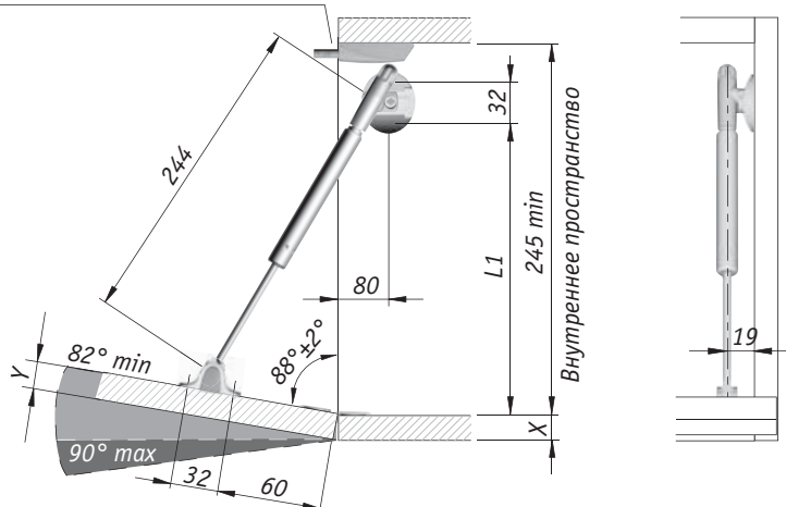
Толкатель K-PUSH TECH средний с магнитом врезной или накладной
