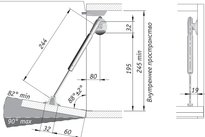
Толкатель K-PUSH TECH короткий с магнитом врезной или накладной
