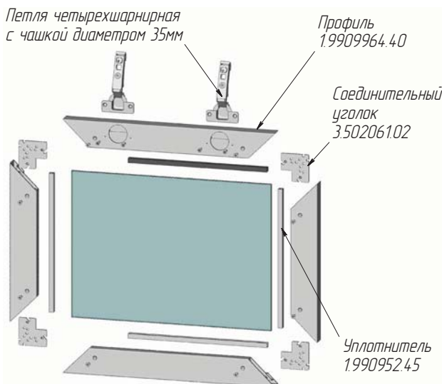
Комплектующие для широкого рамочного профиля
