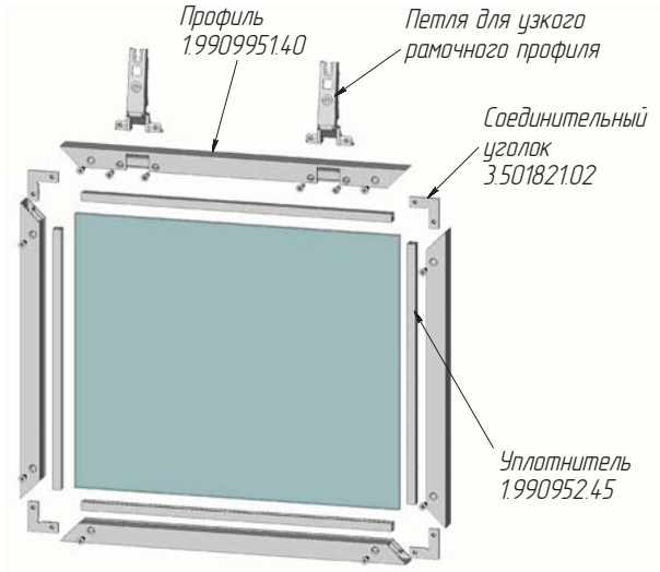
Комплектующие для узкого рамочного профиля
