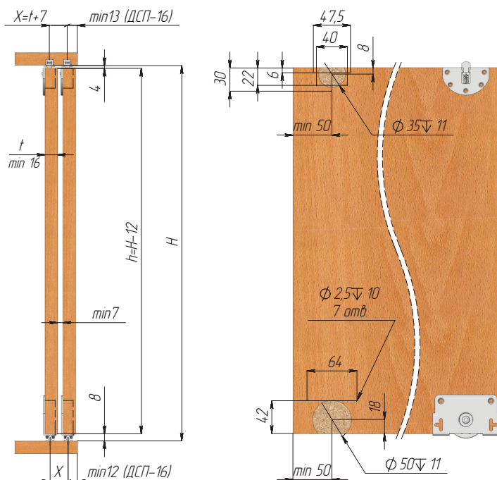
Схема расчетов и сборки с использованием нерегулируемых роликов SKM-60
