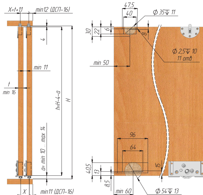
Схема расчетов и сборки с использованием регулируемых роликов SKM-60 AY
