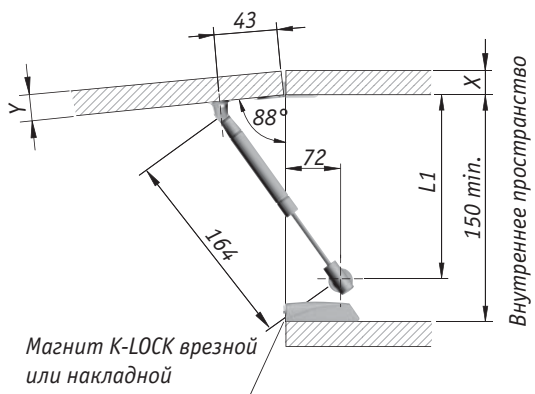
Использование креплений D15
