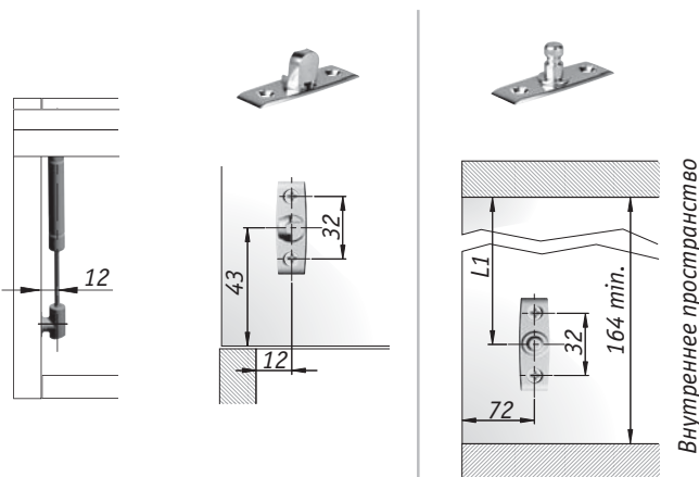
Использование креплений под саморез
