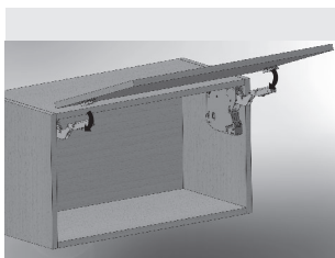
Закрепить механизм саморезами
