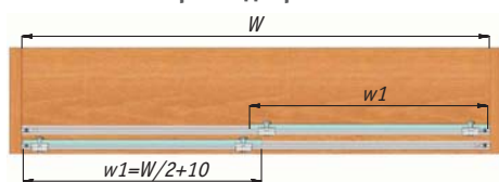
Расчет ширины дверей со стеклом
