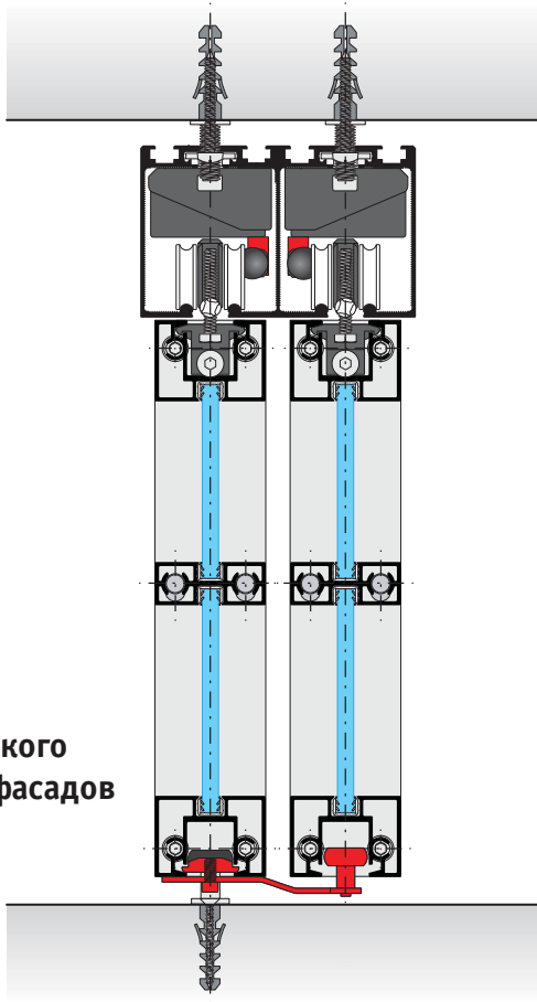
Ролик для телескопического открывания фасадов правый
